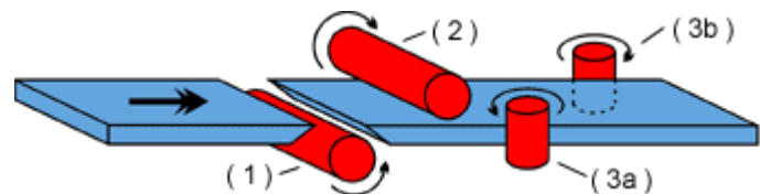
Obrázok 5: Schéma štvorstranného frézovania
